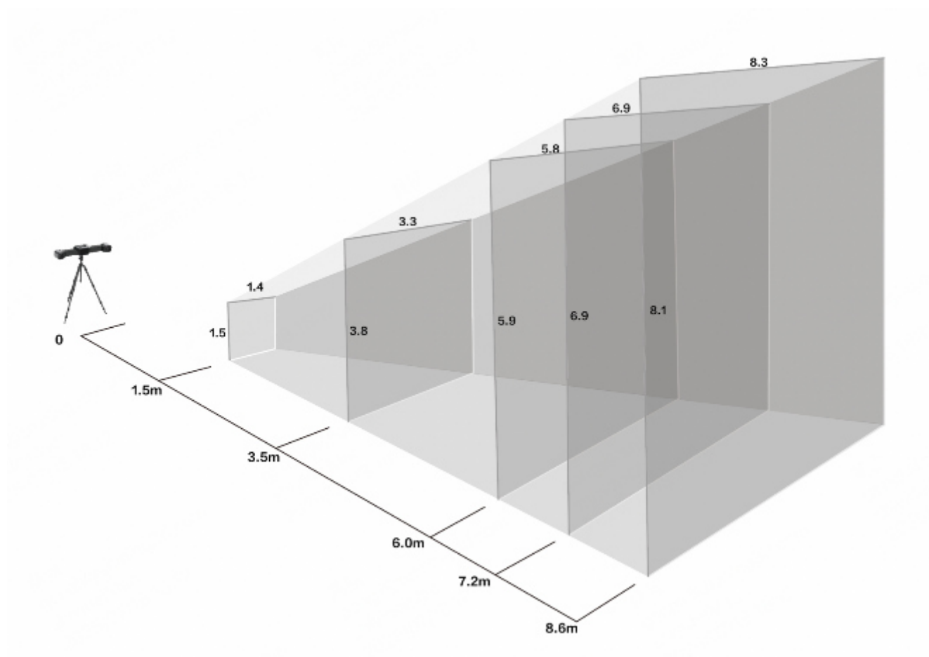
Рисунок 5 – Схема измерительных объёмов модификаций ScanLine TrackerScan Pro W Max (Значения указаны в метрах)
