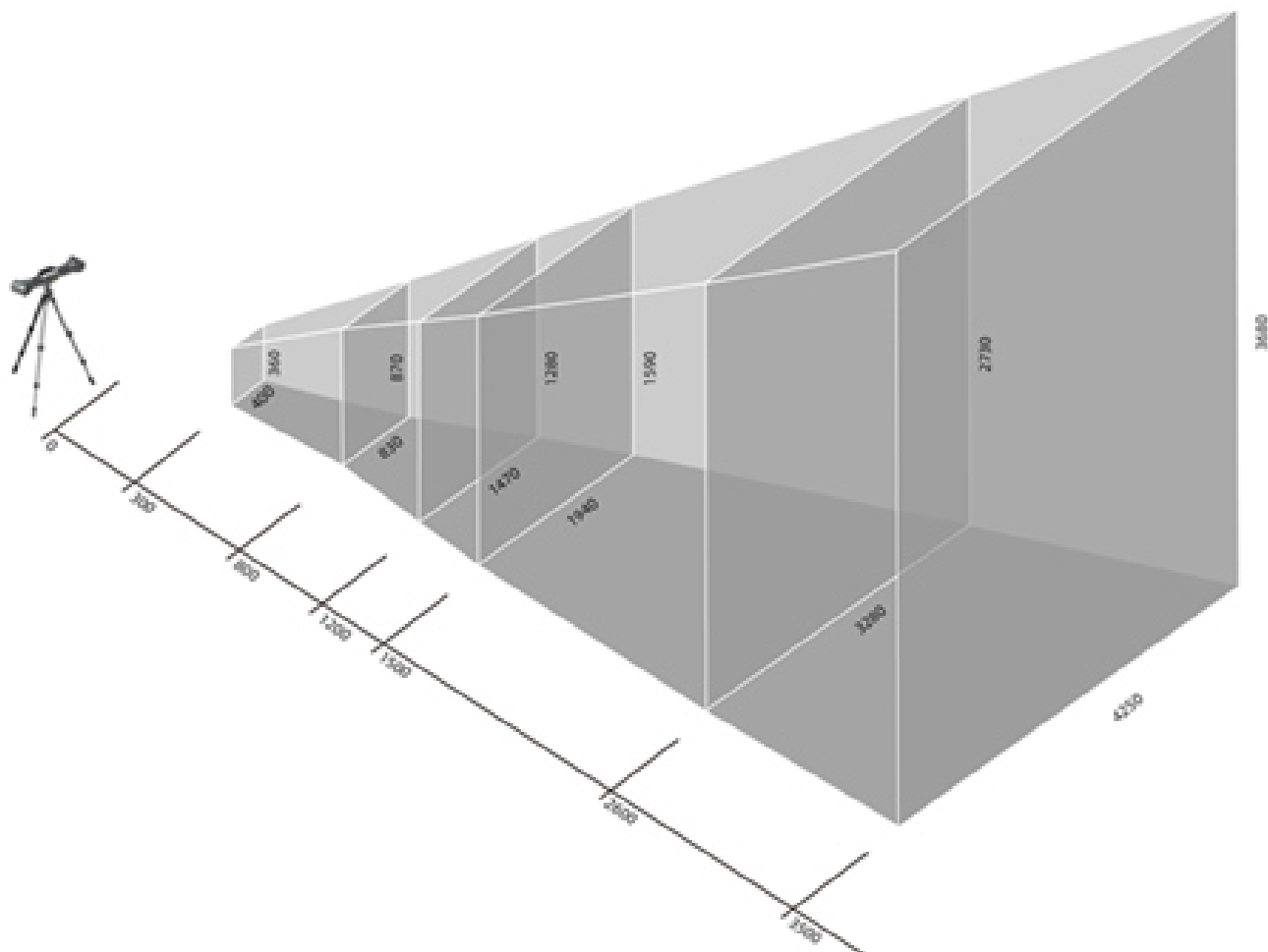
Рисунок 4 – Схема измерительных объёмов модификации ScanLine TrackerScan ProNova, ScanLine TrackerScan ProNova+ (Значения указаны в миллиметрах)
