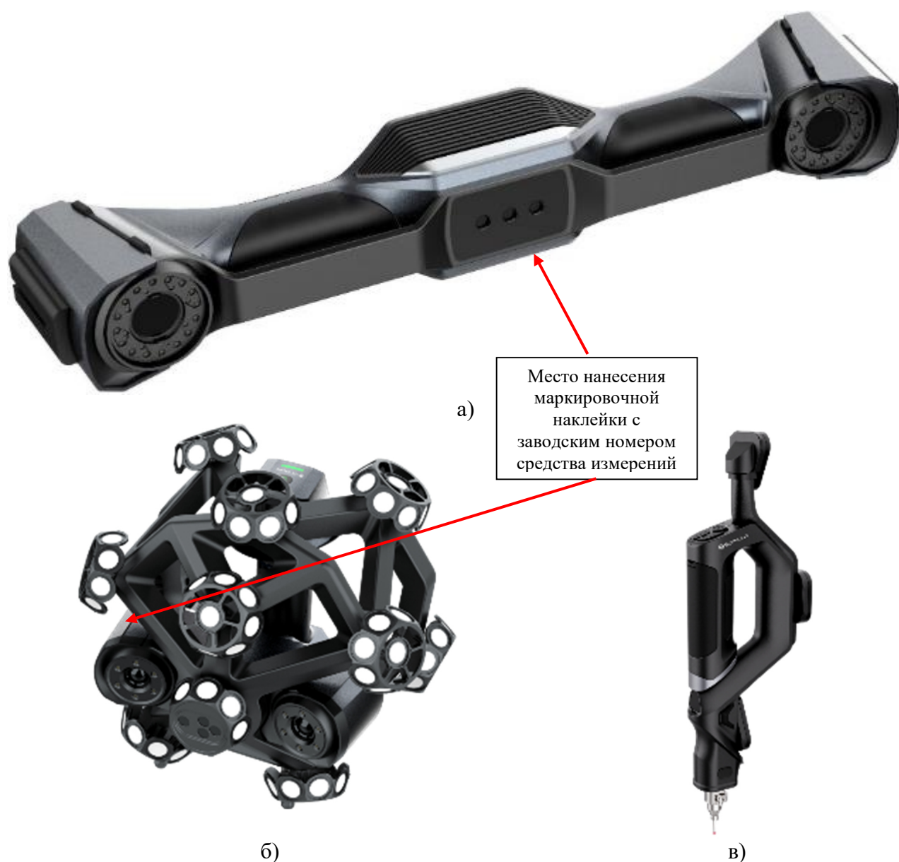
Рисунок 2 – Общий вид основных элементов систем оптических координатно-измерительных ScanLine TrackerScan ProNova, ScanLine TrackerScan ProNova+: а) оптическая система слежения; б) ручной лазерный сканер; в) беспроводной измерительный щуп;
