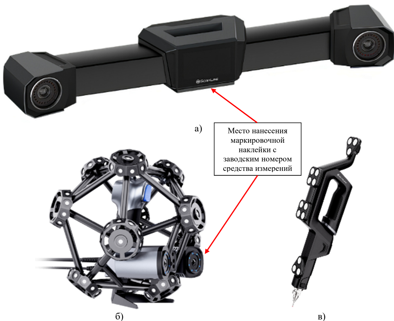
Рисунок 1 – Общий вид основных элементов систем оптических координатно-измерительных ScanLine TrackerScan Pro W Max: а) оптическая система слежения; б) ручной лазерный сканер; в) беспроводной измерительный щуп;
